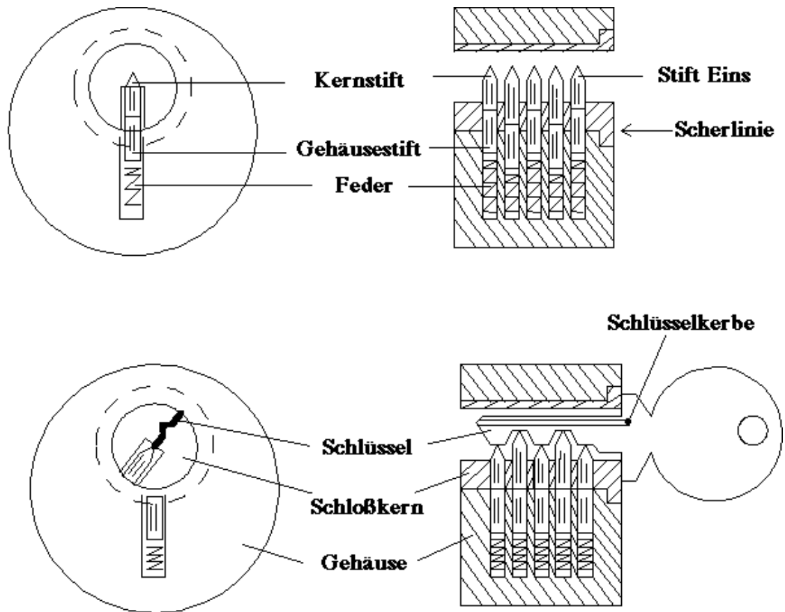
Abbildung 2.1: Arbeitsweise von Stiftzylinder-Schlössern
