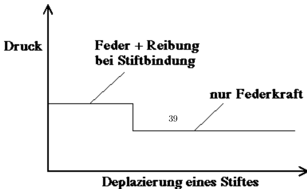
Abbildung 9.3: Dünner Kernstift
