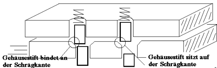
Abbildung 9.6: Der Gehäusestift klemmt in der Schrägfläche
