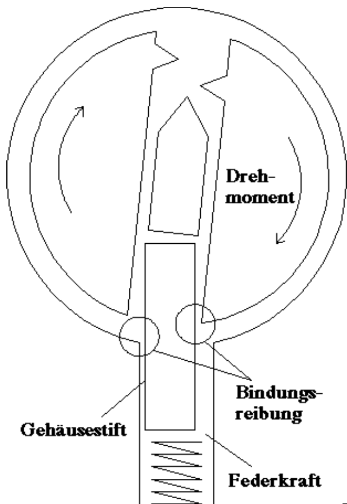
Abbildung 5.2: Der Gehäusestift ist eingeklemmt
