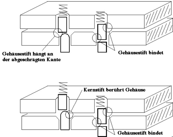
Abbildung 9.4: Abgeschrägte Schloßkernlöcher und abgerundete Kernstifte
