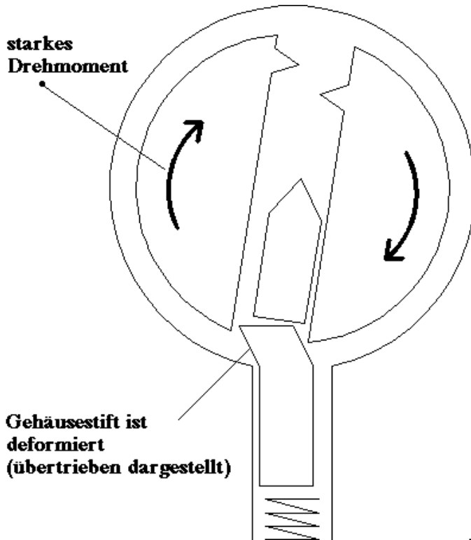
Abbildung 9.2: Der Kernstift hat Bindung bei viel Drehmoment
