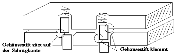
Abbildung 9.5: Der Gehäusestift sitzt auf der Schrägfläche
