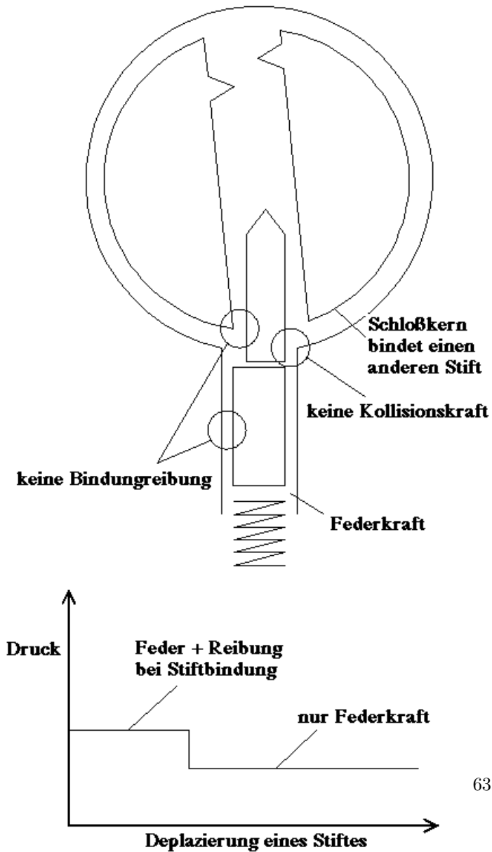
Abbildung 9.3: Dünner Kernstift
