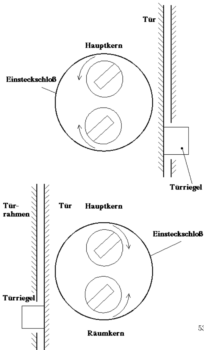
Abbildung 9.1: Die Öffnungsrichtung
