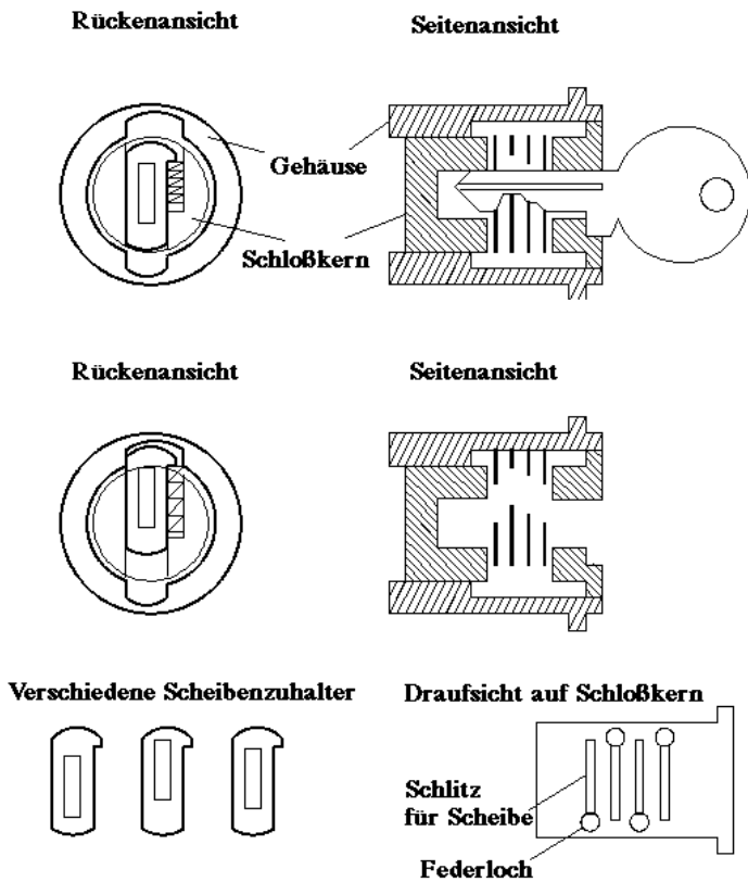
Abbildung 9.10: Arbeitsweise eines Scheibenzuhaltschlosses
