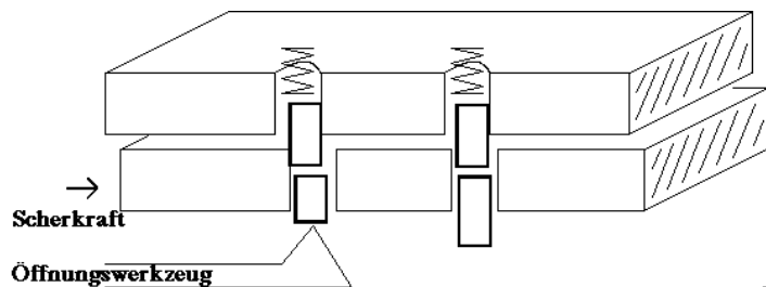
Abbildung 4.2: Das Öffnungswerkzeug drückt den linken Kernstift
