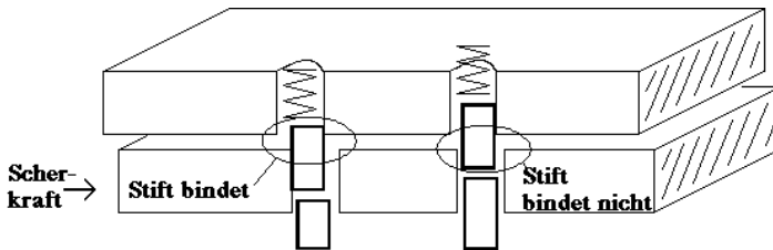
Abbildung 4.1: Einfache Kraft, die den Gehäusestift bindet
