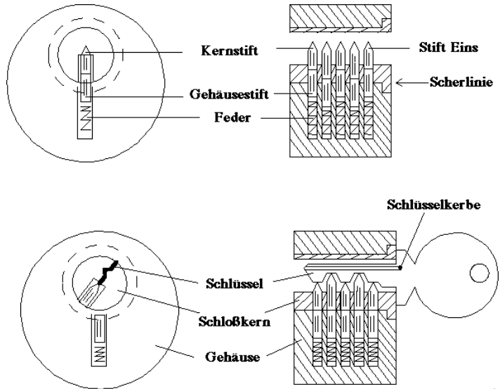
Abbildung 2.1: Arbeitsweise von Stiftzählungsschlössern
