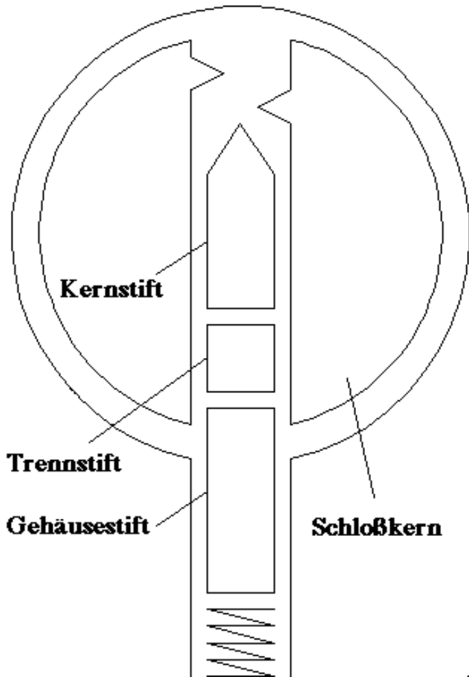
Abbildung 9.8: Trennstifte in der Stiftsäule
