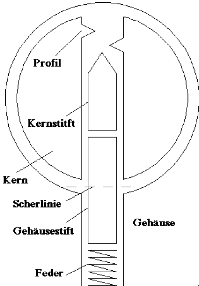
Abbildung 5.1: Das Stift-Säulen-Modell
