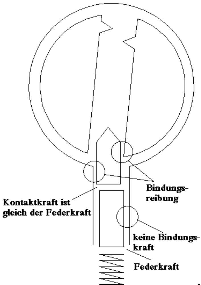
Abbildung 5.4: Der Kernstift dringt in das Gehäuse ein
