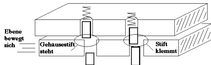
Abbildung 4.3: Der Kernstift fällt auf seinen Stifthalter zurück
